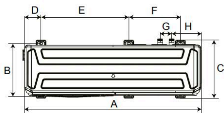
4/6 kW (unité : mm)
