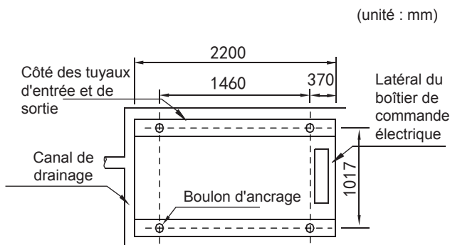
III. 6-6 Vue du dessus du schéma des dimensions de l'installation de 110 kW, 140 kW
