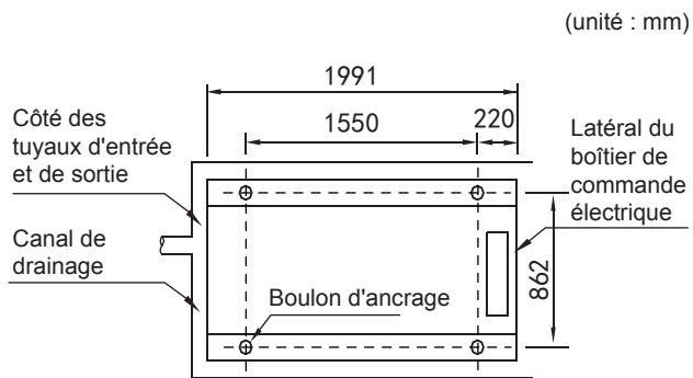
III. 6-5 Vue du dessus du schéma des dimensions de l'installation de 50 kW, 65 kW, 75 kW
