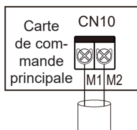
Connexion à l'ODU M1M2 (HyperLink)
